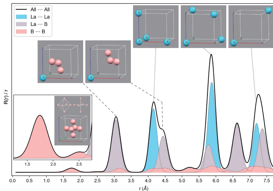
圖二 理論模擬原子成對分佈函數， \text{LaB}_6 (SRM 660c), (La...La, La...B, B...B)。
